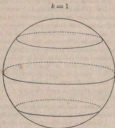
FIG. 5.* — (Sfera).
