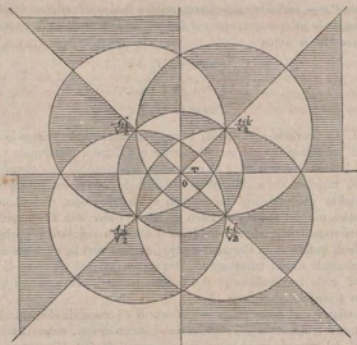
FIG. 9.° — (Rete ottaedrica).
